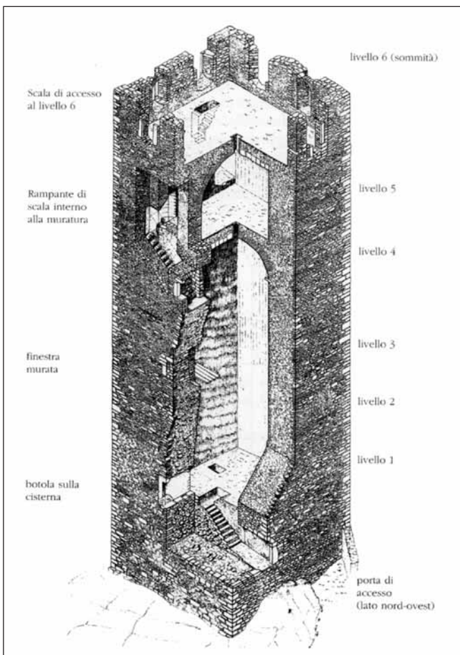
Spaccato assonometrico della torre
